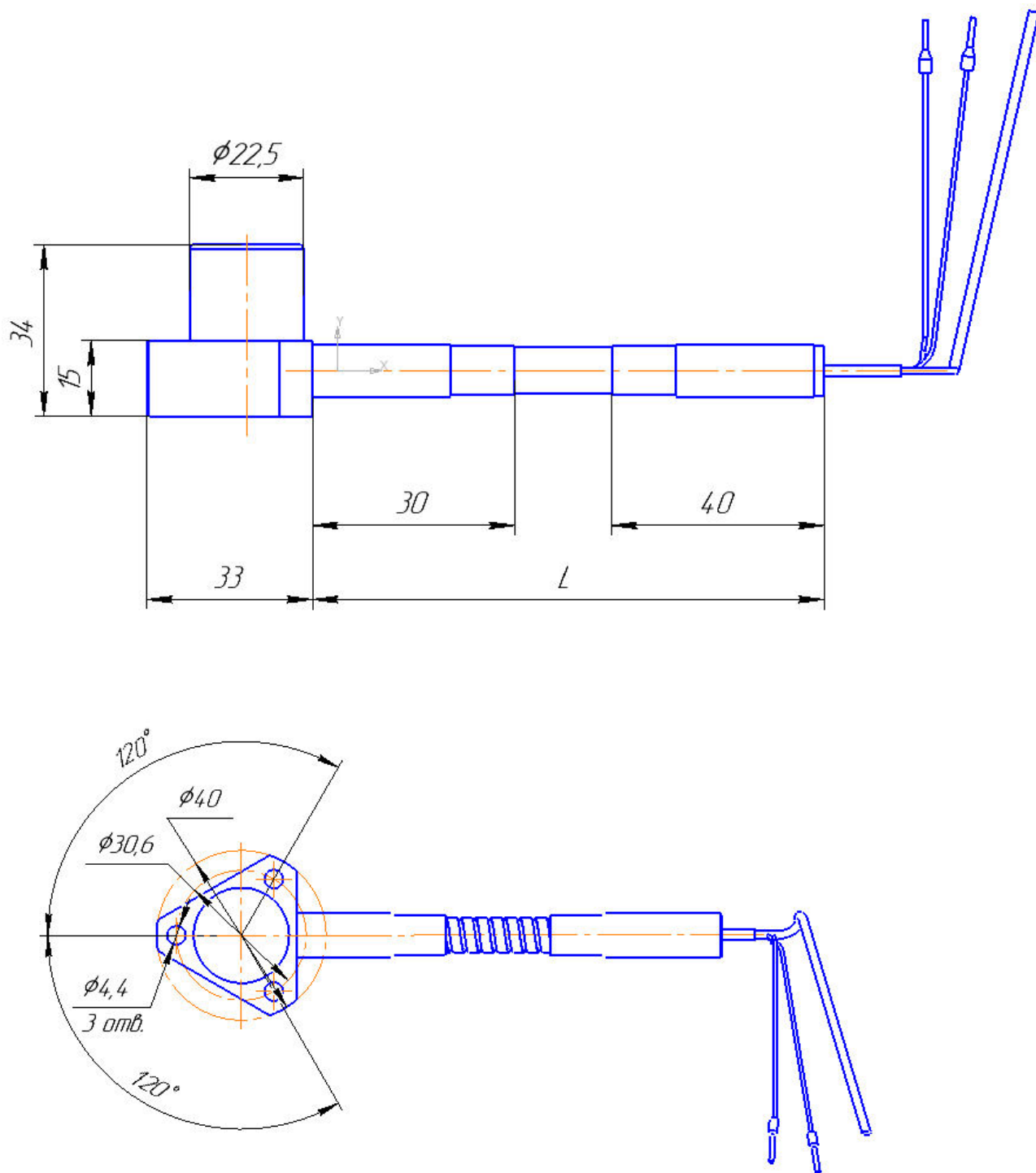
Габаритный чертеж вибропреобразователя ВК-310VX (вариант с боковым расположением кабеля).
