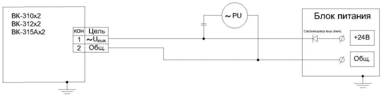
Рис 7. Типовые схемы подключения вибропреобразователей (на рисунке: РА, РU-амперметр, вольтметр соответственно)
