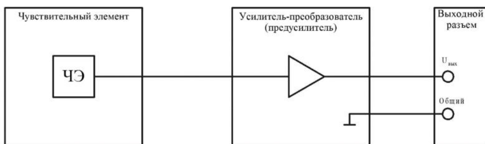
Рис. 1 Структурная схема преобразователей ВК-310х2, ВК-312х2, ВК-315Ах2
