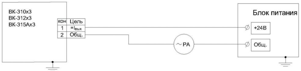
Рис 7. Типовые схемы подключения вибропреобразователей (на рисунке: РА, РU-амперметр, вольтметр соответственно)
